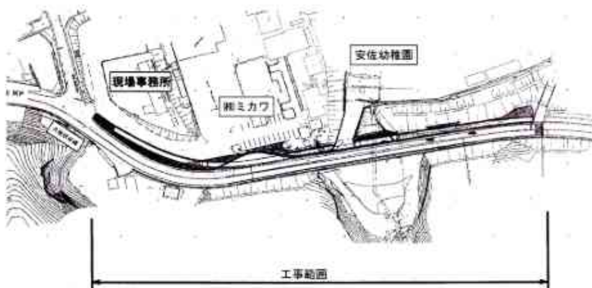
工事現場位置図(詳細)
